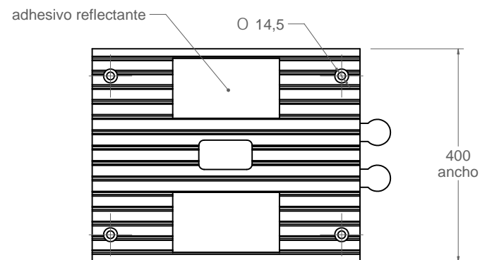
vista en planta 1:10
