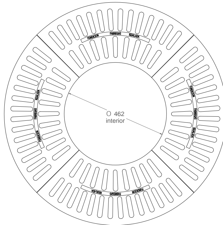
vista en planta 1:10
