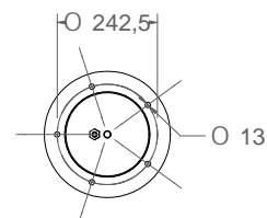
CORTE B-B 1:20
