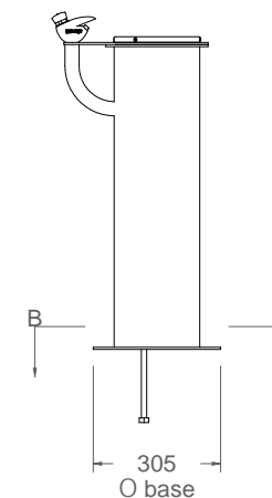
vista lateral 1:20
