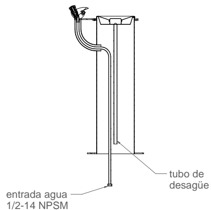
CORTE A-A 1:20
