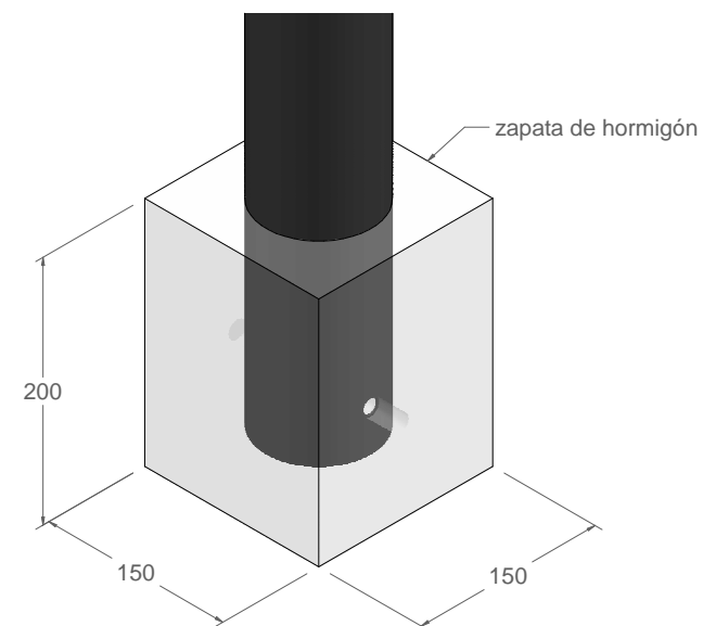
detalle anclaje 1:5
