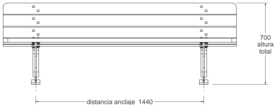
vista alzado 1:20
