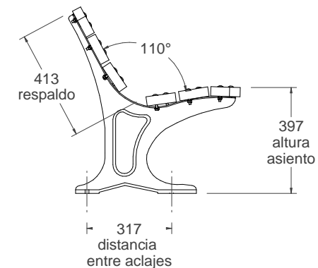
vista lateral 1:20
