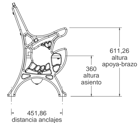
vista lateral 1:20
