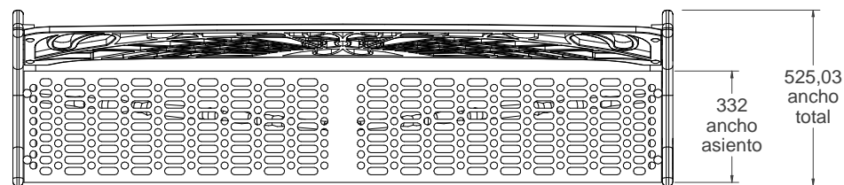
vista en planta 1:20
