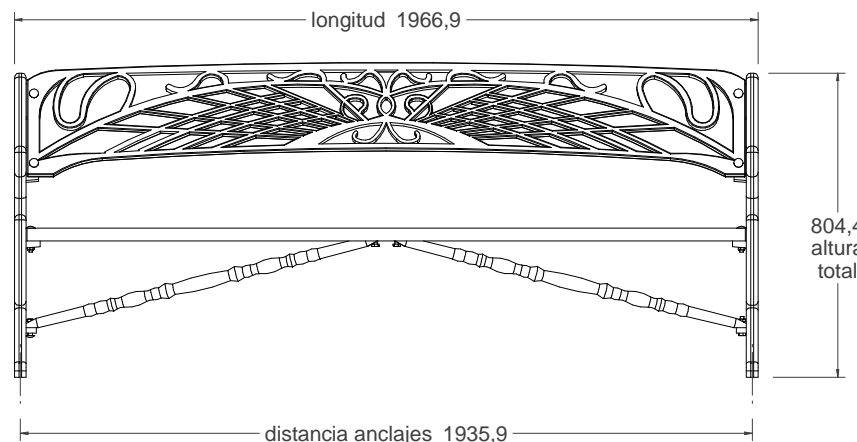
vista alzado 1:20
