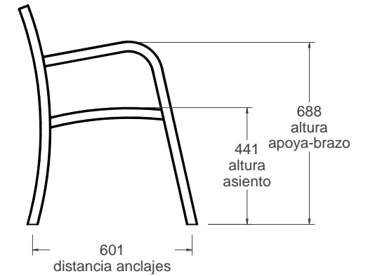
vista lateral 1:20
