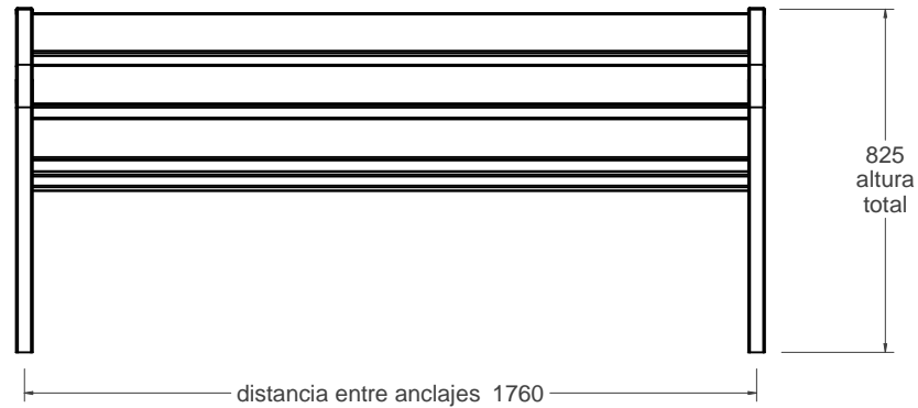
vista alzado 1:20
