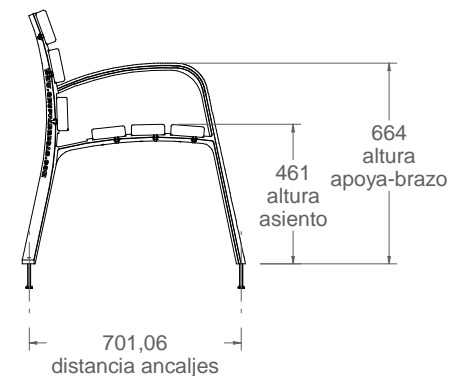
vista lateral 1:25
