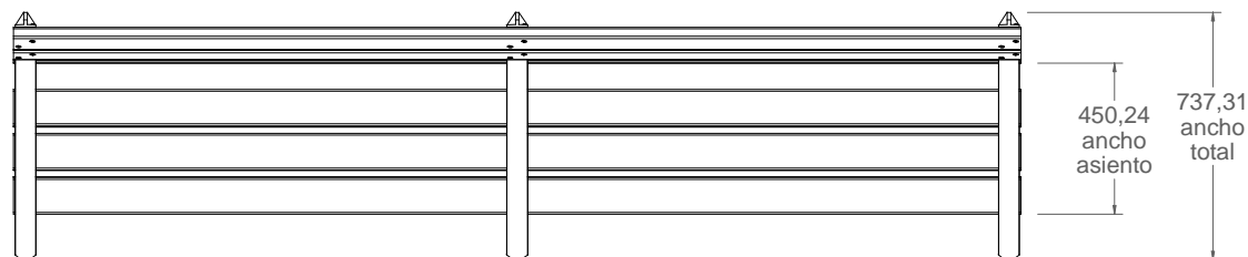
vista en planta 1:25
