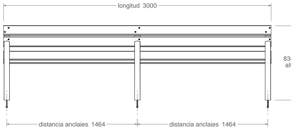
vista alzado 1:25
