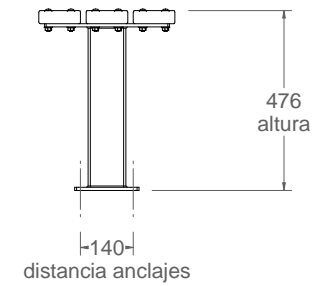
vista lateral 1:20
