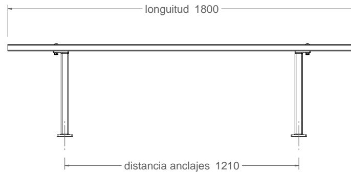
vista alzado 1:20
