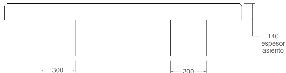
vista alzado 1:20
