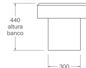
vista lateral 1:20
