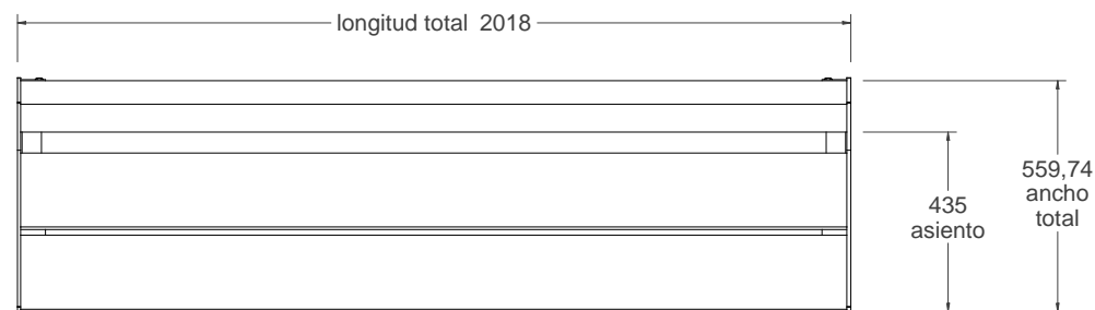
vista en planta 1:20
