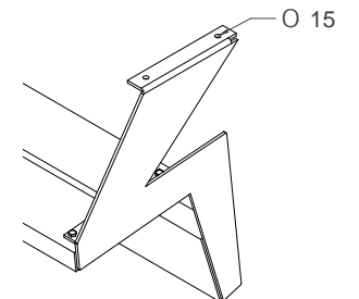
detalle anclaje 1:20
