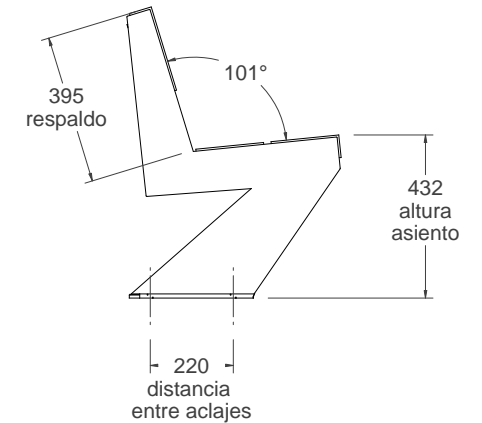
vista lateral 1:20
