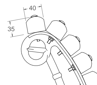
DETALLE A
