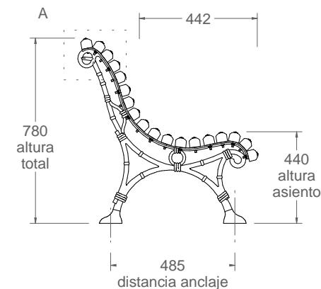
vista lateral 1:20
