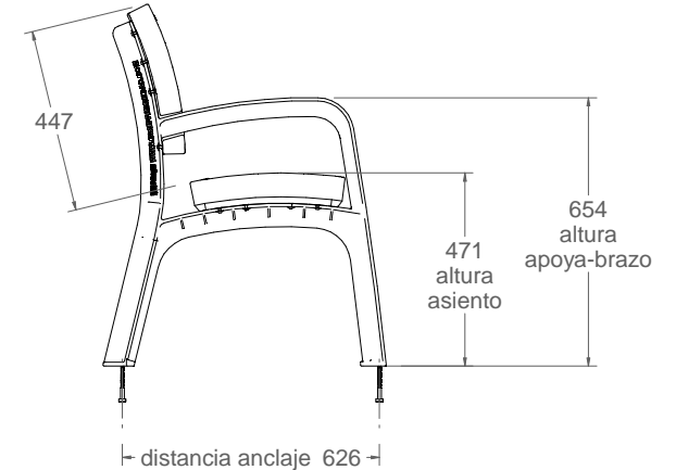
vista lateral 1:20
