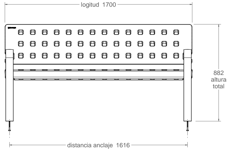
vista frontal 1:20
